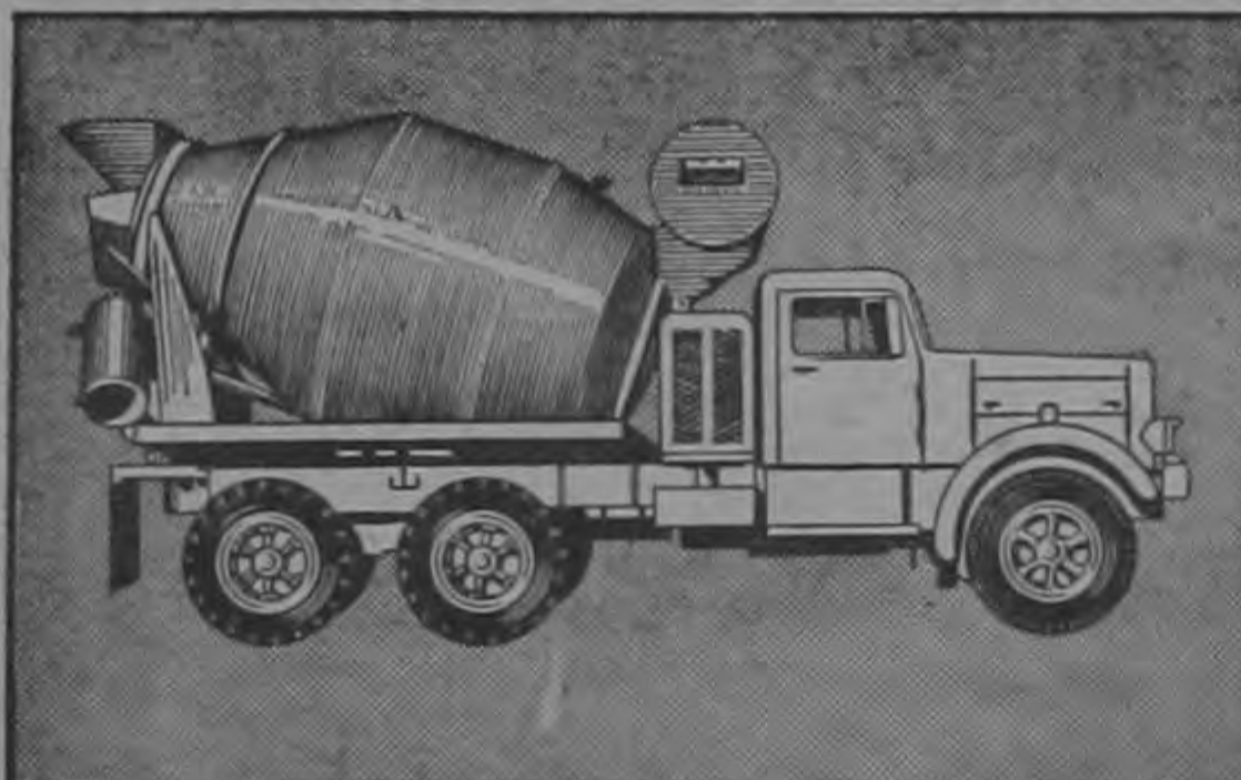
Robusta Hormigonera para Camiones, diseñada para la más variada clasificación de especificaciones de hormigón, característica que rinde mayores utilidades. El tambor de "bajo asentamiento" tiene una inclinación de 18 grados, para asegurar máxima capacidad de acarreo, y una boca de descarga de 44 pulgadas.
