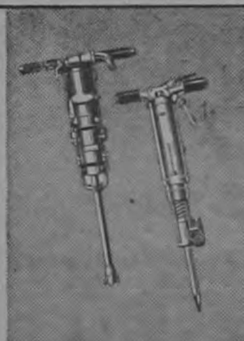
Las Herramientas Neumáticas son de gran durabilidad integral y vienen en una amplia variedad de diseños para diferentes trabajos. Ilustramos aquí la perforadora para roca WS-55 y el martillo rompedor WB-82.
