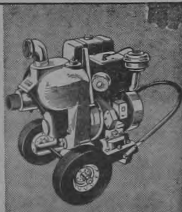
La Bomba Portátil Autocebante puede llevarse fácilmente de un trabajo a otro. Las de aluminio pueden obtenerse en tamaños de 1-1/2 pulg.; las otras, en tamaños de 4, 6 y 8 pulgadas, y en capacidades hasta de 125.000 galones por hora.
