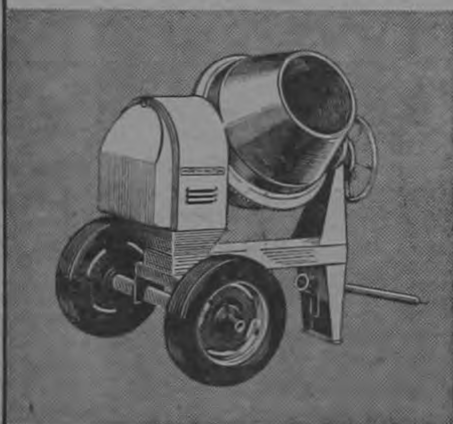
Hormigonera Portátil, eficiente y económica para mezclar en la obra. En gran variedad de modelos, desde 3-1/2 pies cúbicos con basculador de descarga lateral, hasta de 16 pies cúbicos con descarga basculante de costado y hacia atrás.
